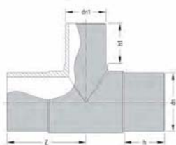
TE REDUCIDA 90°
