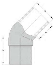
CODO 45°
